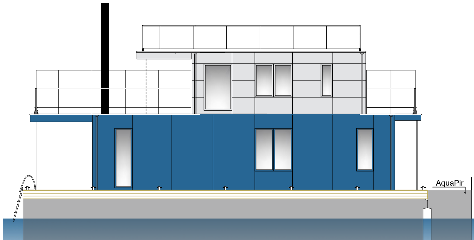
Styrbord fasad SKALA 1:100
