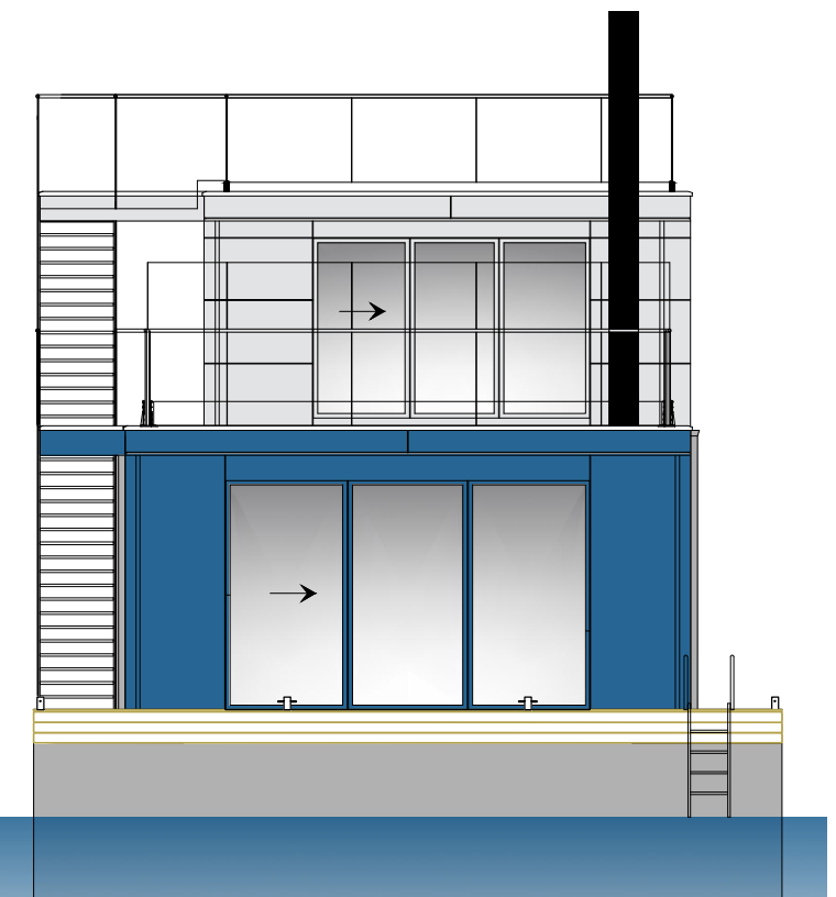
Terrass fasad SKALA 1:100
