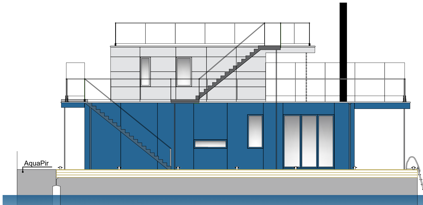
Babord fasad SKALA 1:100
