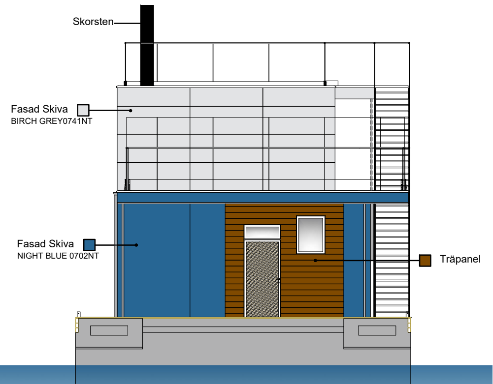
Entré fasad SKALA 1:100
