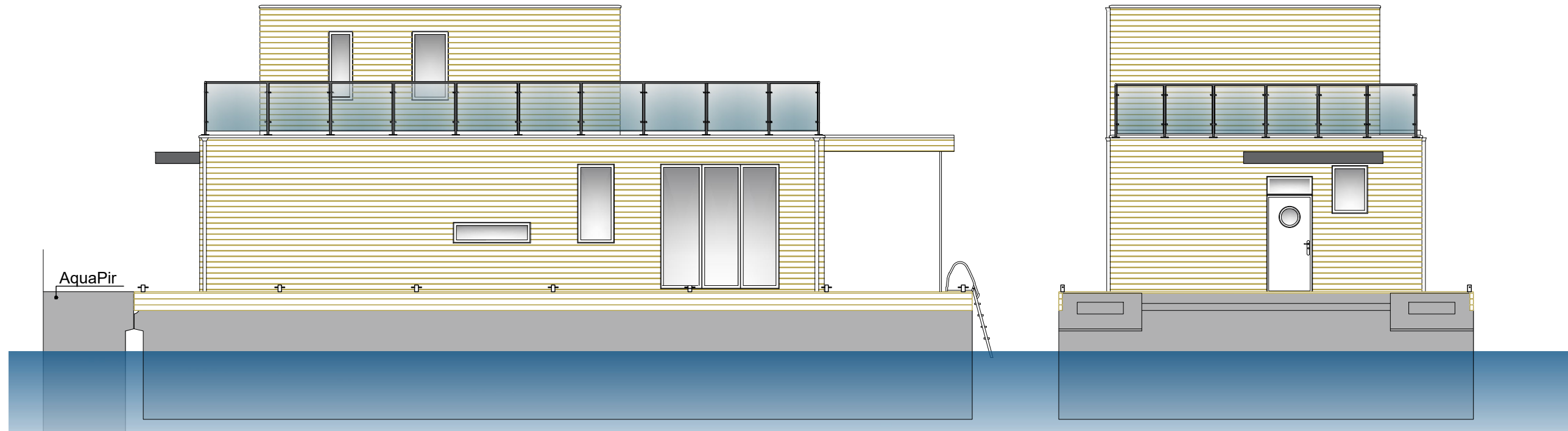
Babord fasad SKALA 1:100
