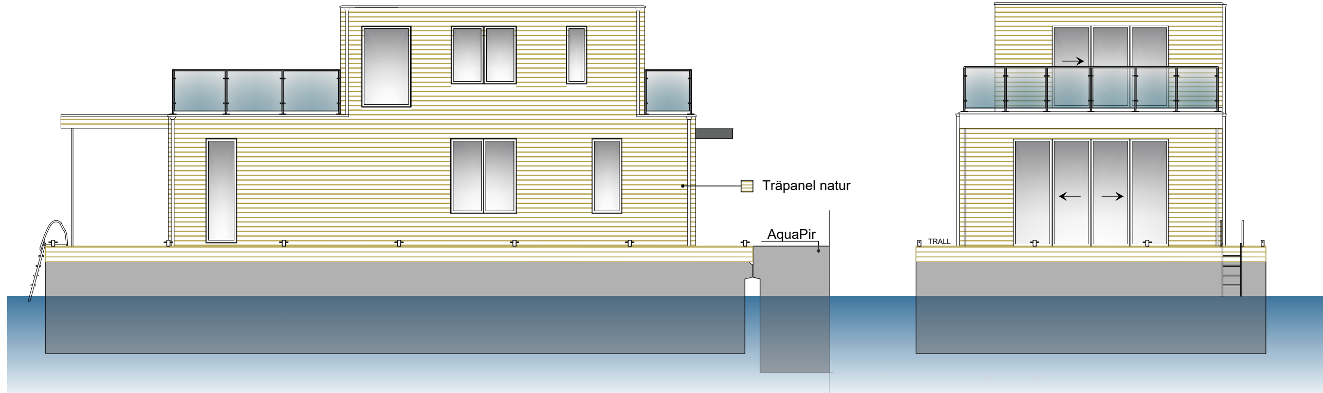
Stybord fasad SKALA 1:100
