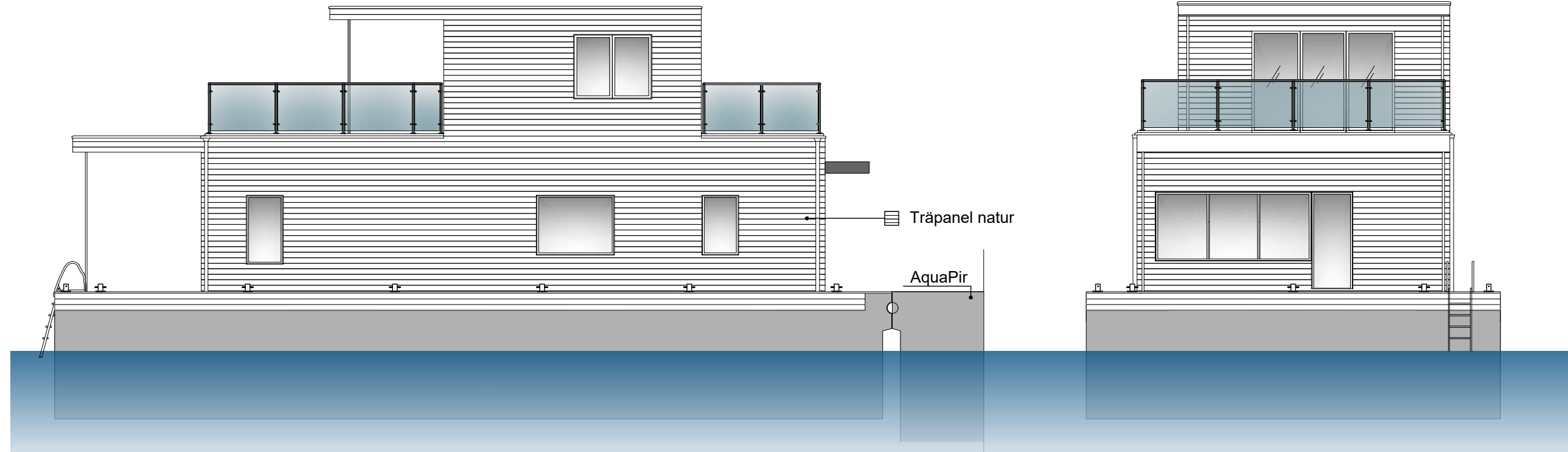
Stybord fasad SKALA 1:100
