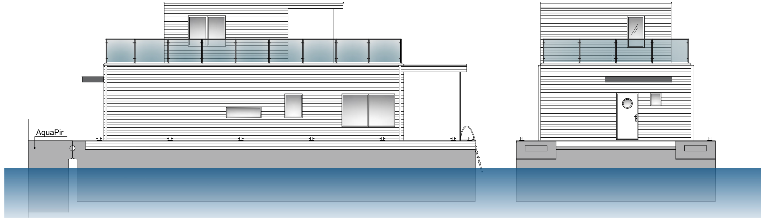
Babord fasad SKALA 1:100
