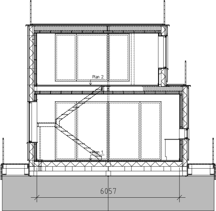
Tvärsektion, cross section
