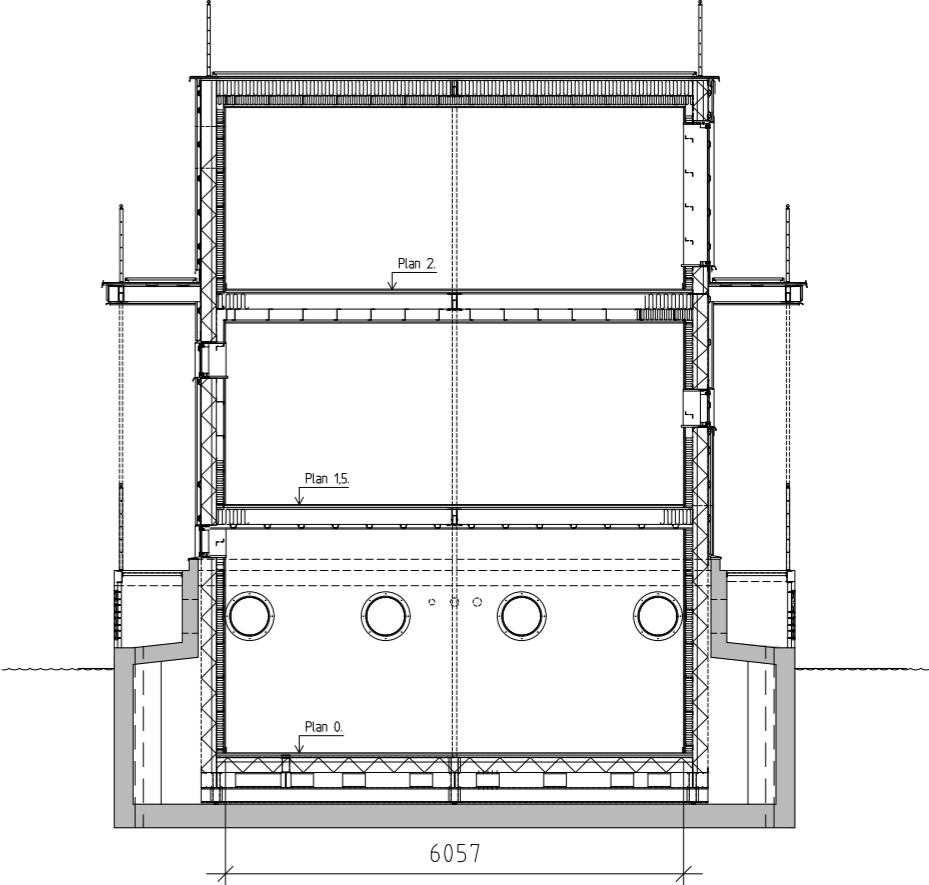
Tvärsektion, cross section
