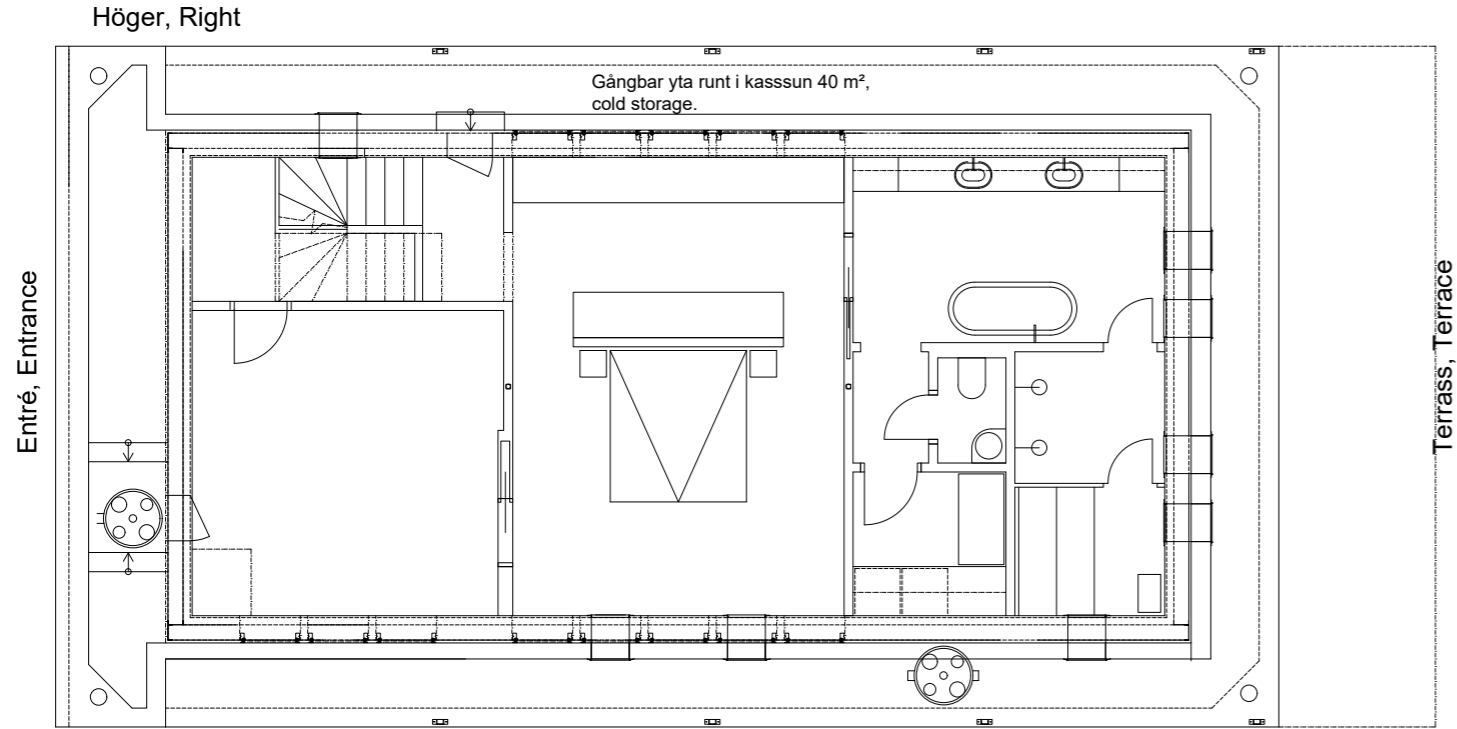
Vänster, Left Plan 0, Kassunplan 78m 2
