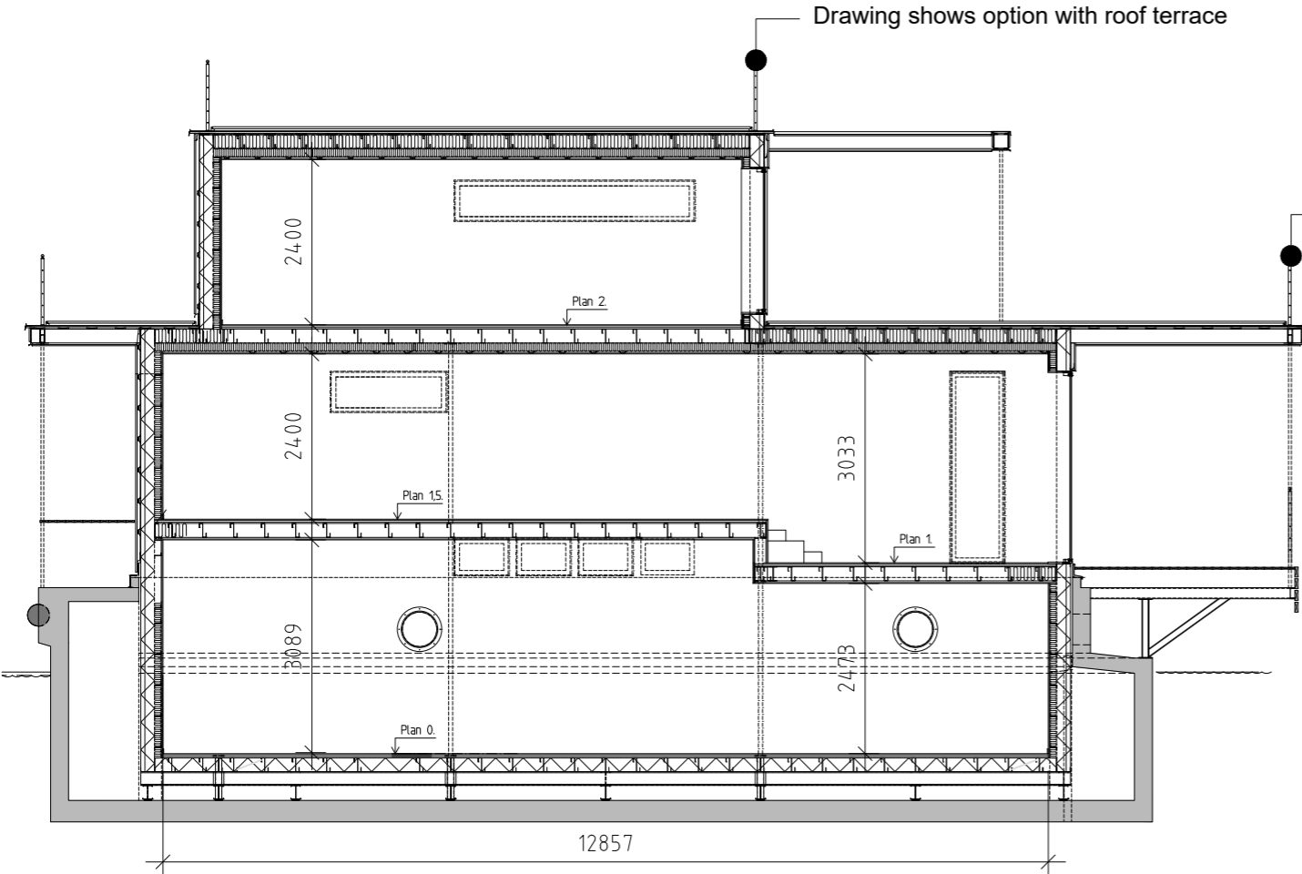
Längdsektion, longitudinal section
